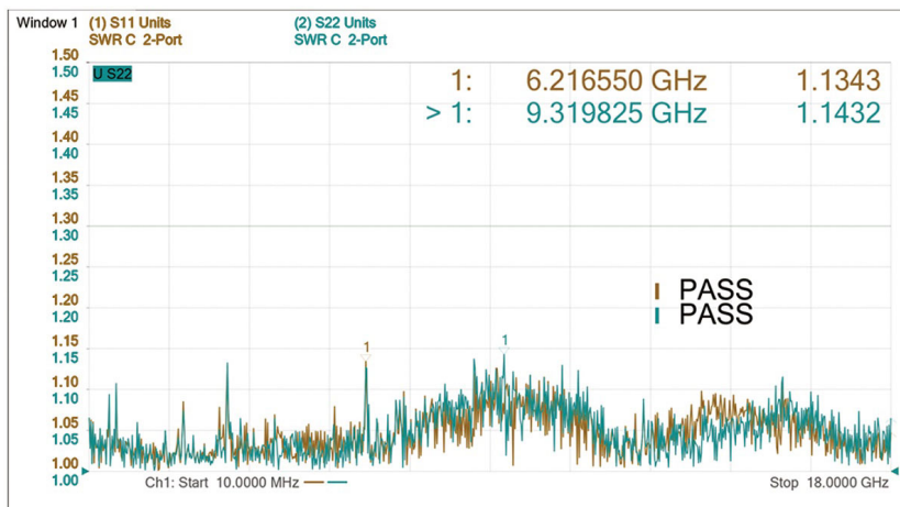
VSWR测试曲线(A20-07-07-3M/VA2)
