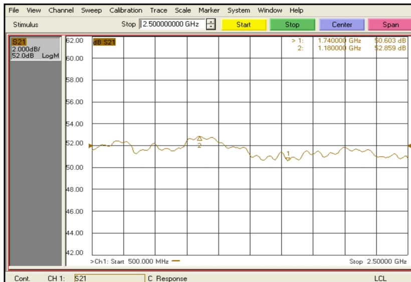
增益 S21 (Pin= 0 dBm, 连续波, 负载驻波 \leq 1.2 , 25°C), 增益平坦度, 参考曲线
