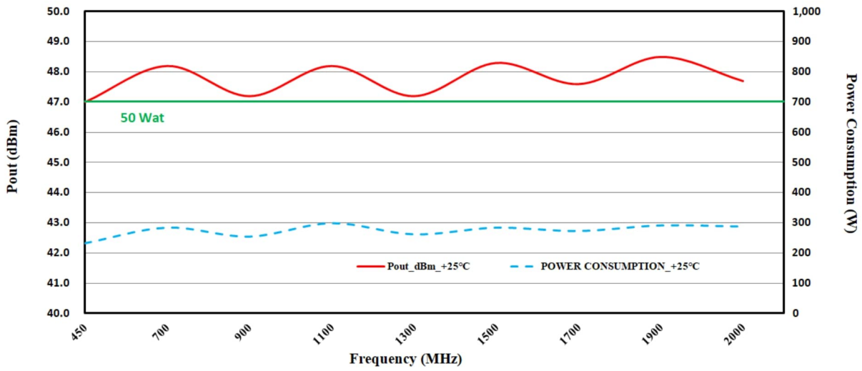
饱和功率 & 功耗 (连续波, 负载驻波 \leq 1.2 , 25°C)
