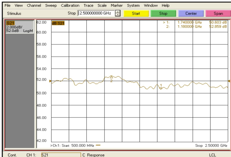
增益 S21 (Pin= 0 dBm, 连续波, 负载驻波 \leq 1.2 , 25°C), 增益平坦度, 参考曲线
